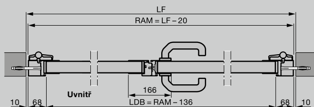
Dvoukřídlové vedlejší dveře s hliníkovou blokovou zárubní, profil typu 2 Montáž v otvoru
